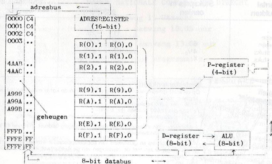
fig. 4 Processor met geheugen.
